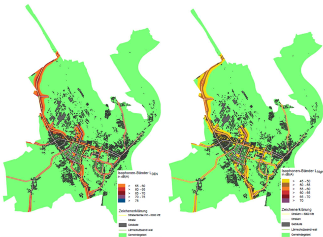
Eisenhüttenstadt: Lärmkarten L_{DEN} und L_{Night} (Quelle: LUGV)
